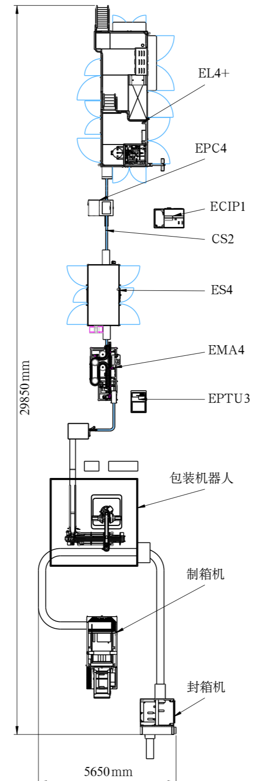
灌装线平面示例
